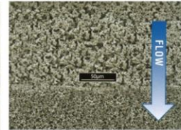
尼龍除菌膜打褶設計及漸密式結構，能提供卓越的過濾效能。
